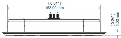
俯视图
